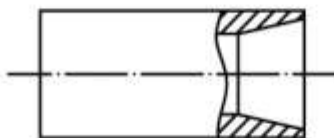
Innen-Taper (verschiedene Winkel und gleichzeitig Planen möglich)
