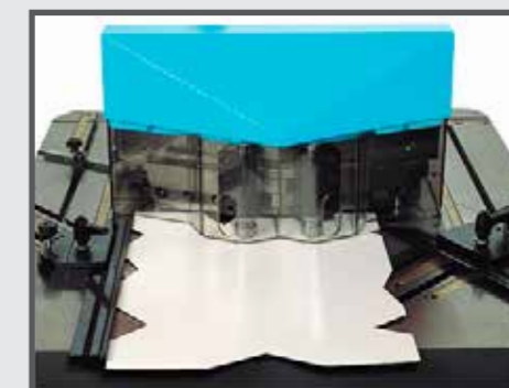
Arbeitstisch mit graviertem Lineal und Anschläge mit Nonius, mehrere Positionen fixierbar.
